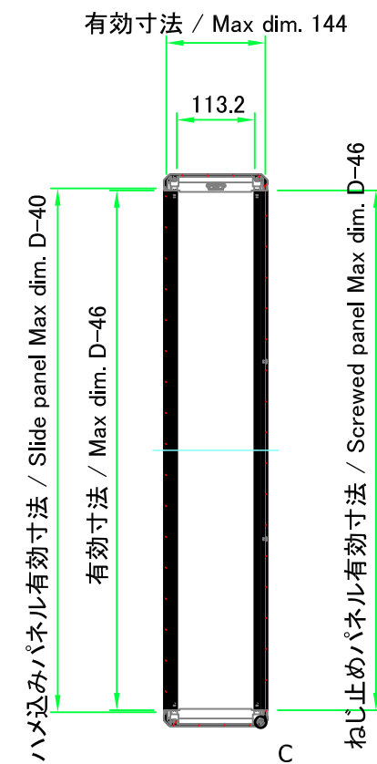
B-B ( 1 : 10 )
